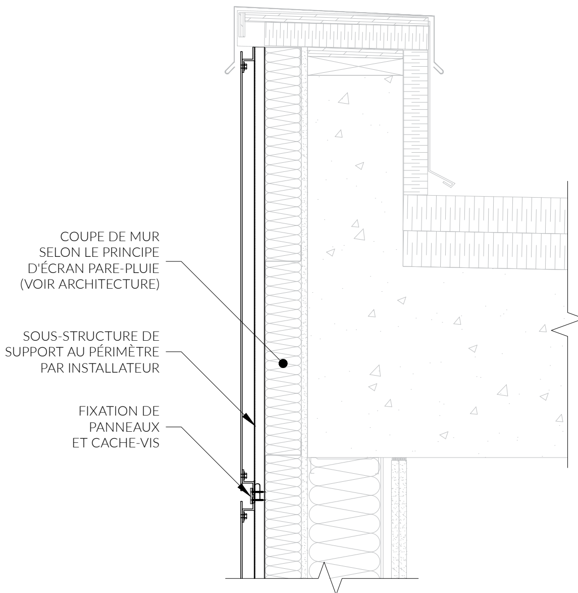
01 TÊTE MUR/PARAPET ÉCHELLE 1:8
