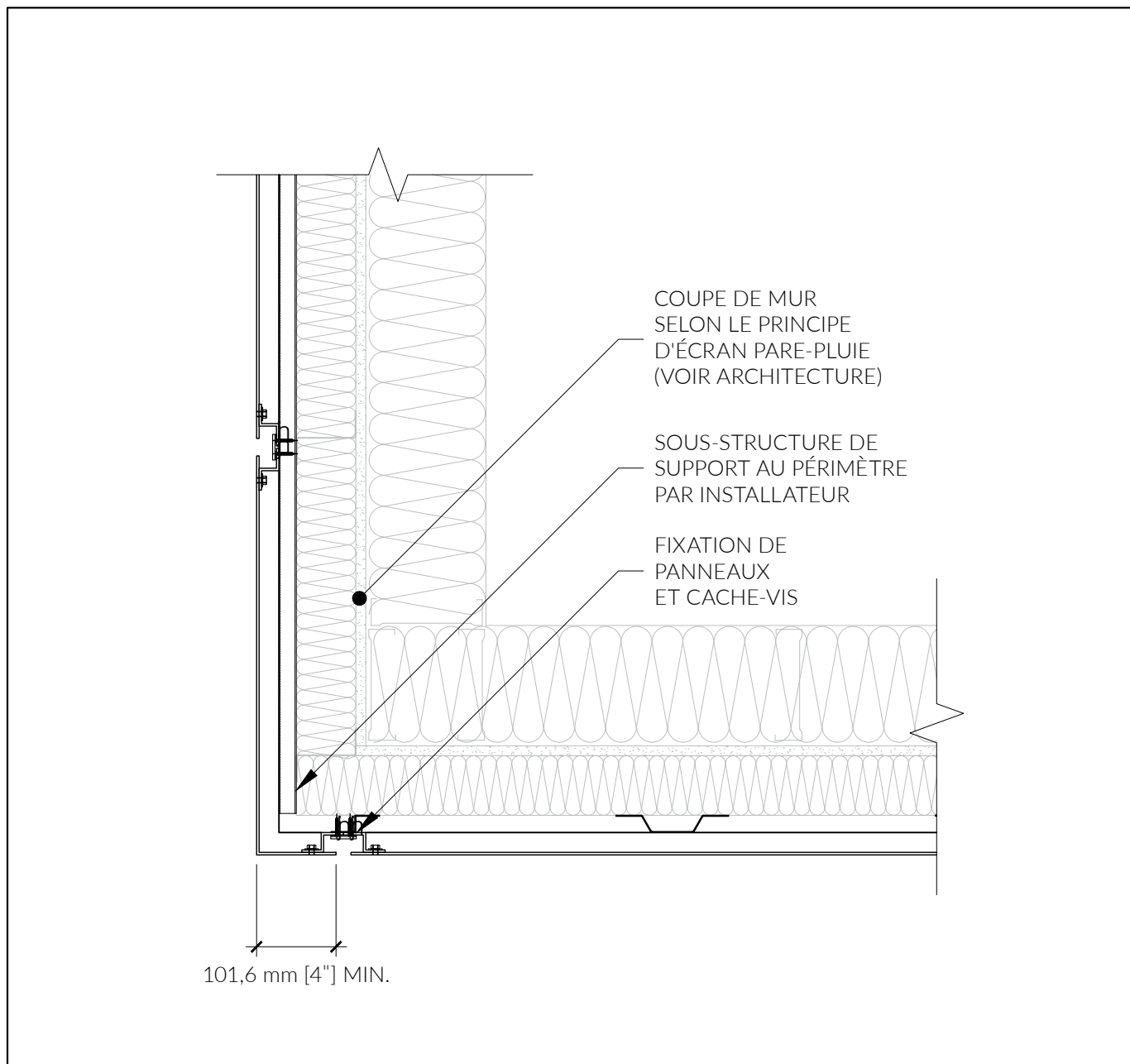
13a SEUIL MUR ET SOFFITE SH-01 ÉCHELLE 1:8
