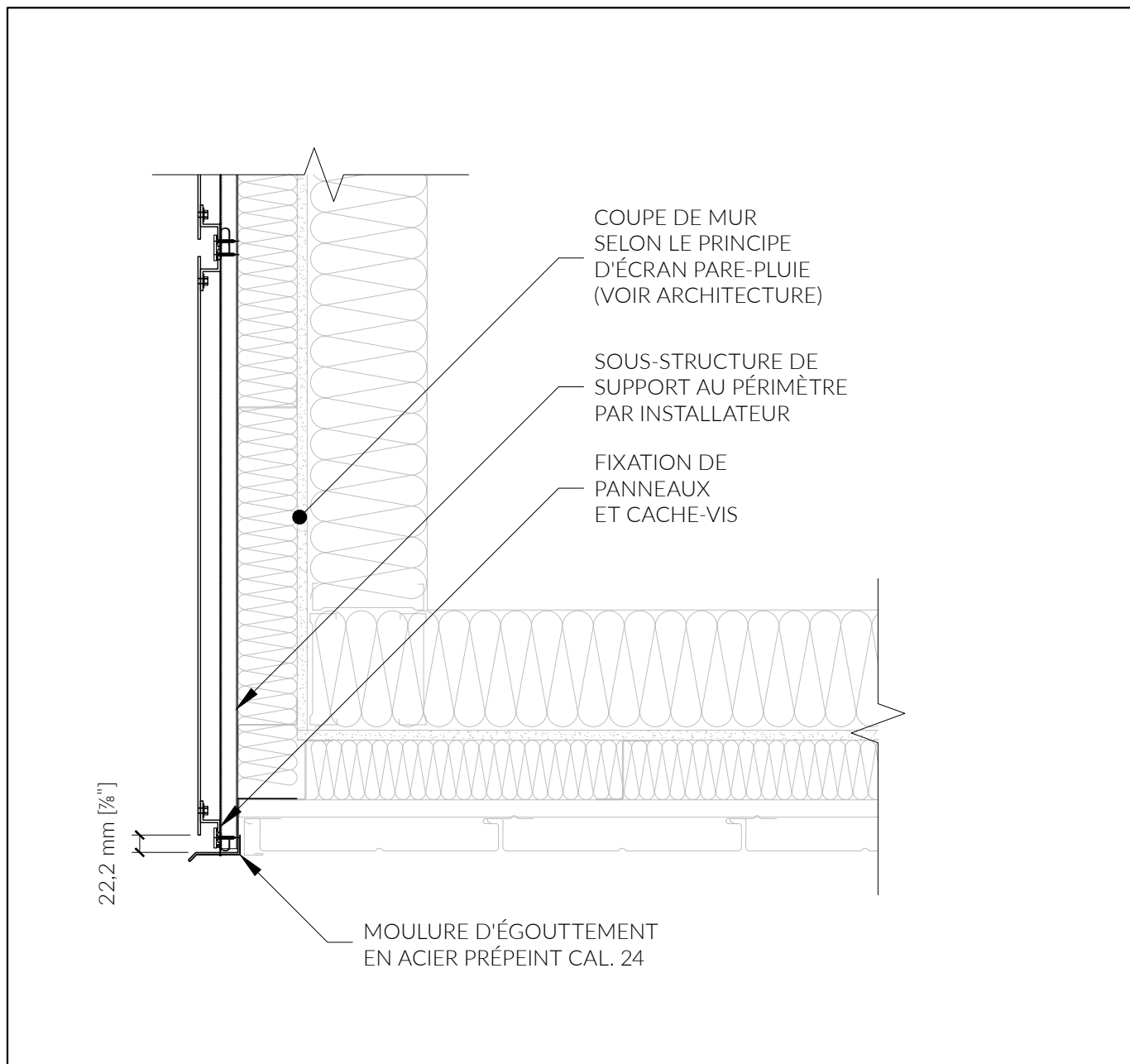
13b SEUIL MUR ET SOFFITE AUTRE ÉCHELLE 1:8
