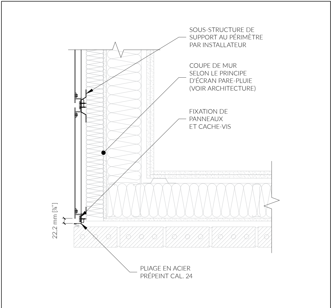
21 FIN DE MUR/TRANSITION ÉCHELLE 1:8
